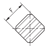
Corte AA (Quadrado de arraste)
