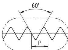
Detalhe do perfil da rosca
